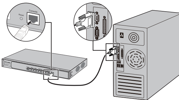
图3-2 Console端口连接示意图
